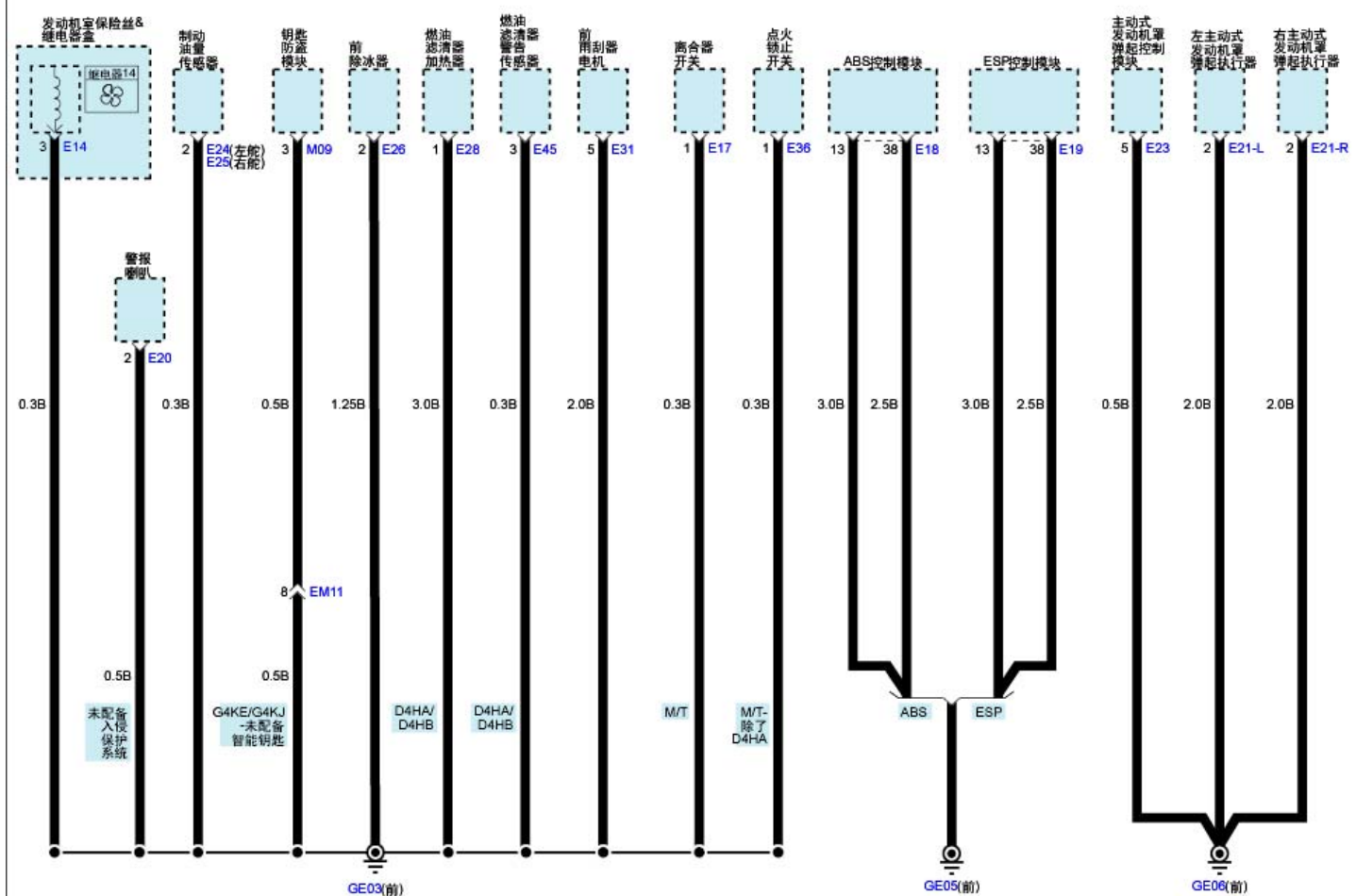
搭铁分布(7)
